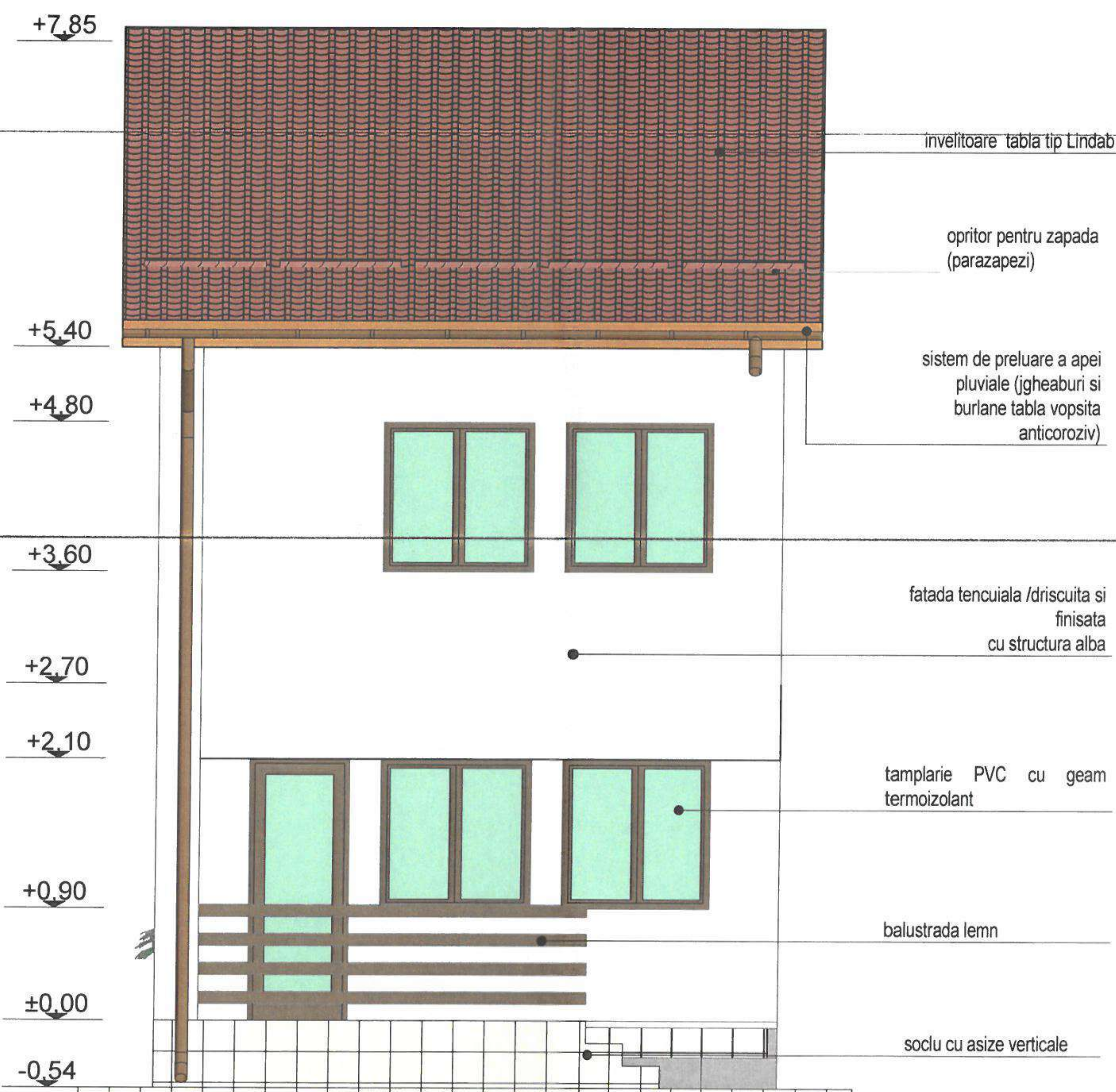
FATADA POSTERIOARA SC 1/50
